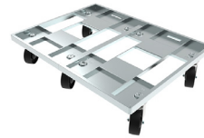
BODENROLLER FÜR KLT 800 X 600, MIT 5 LENKROLLEN
