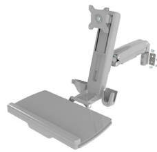
MONITOR ARBEITSPLATZ SIT / STAND 4 ACHSEN, PROFILBEFESTIGUNG (SET)
